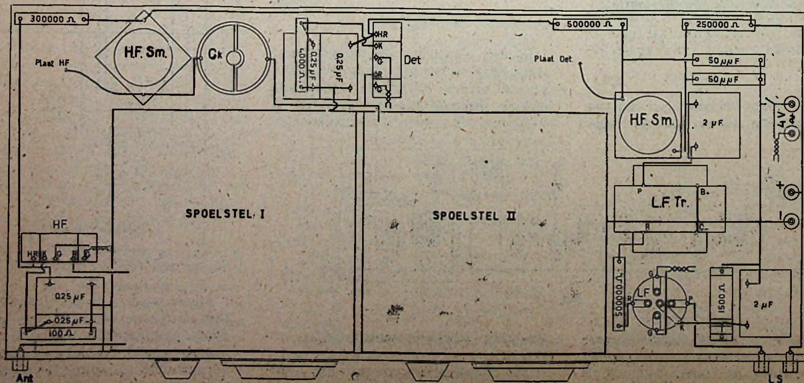
Fig. 5. Bouwteekening en ontwerp G. J. Eschauzier; \frac{1}{3} ware grootte.
